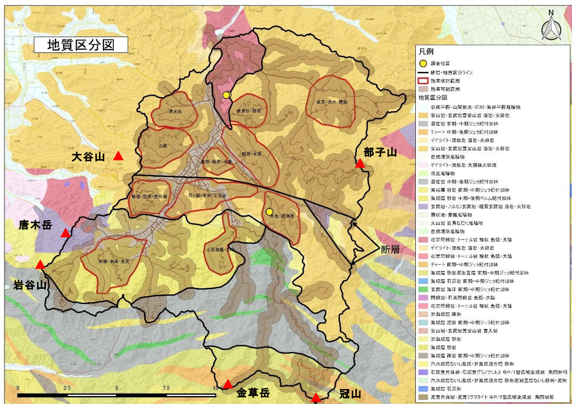
図 1. 地質区分図
