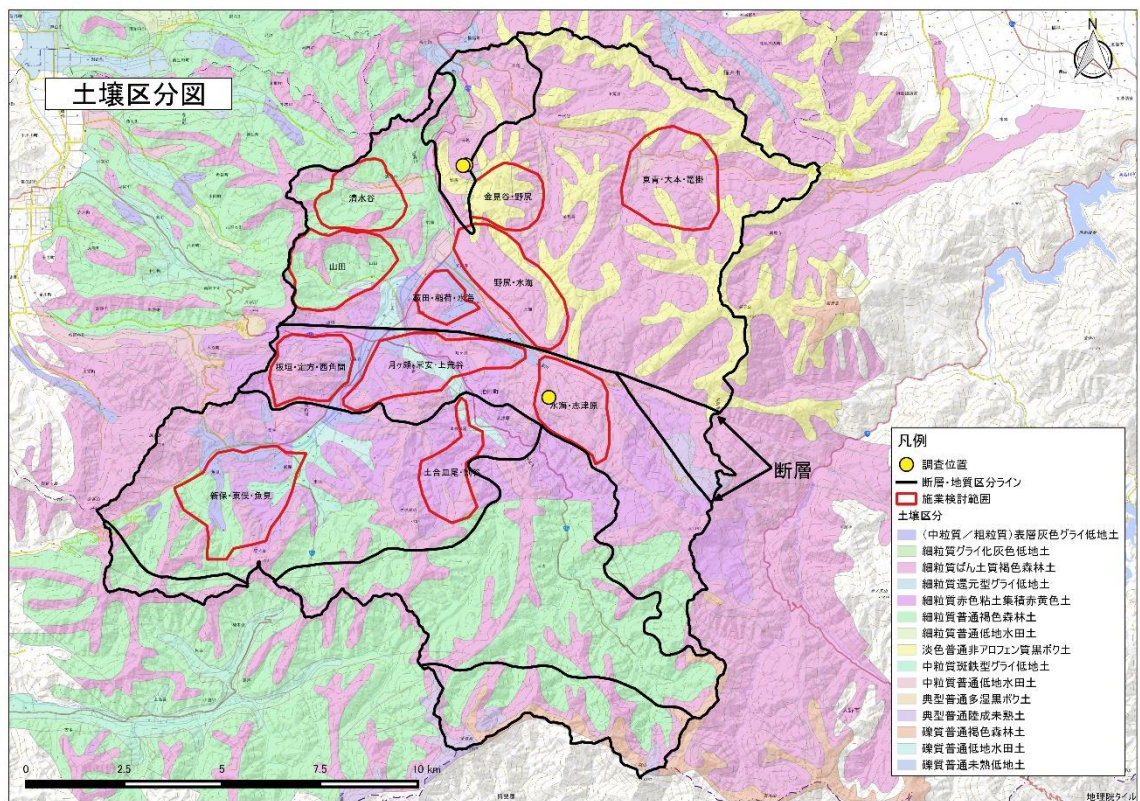
図 2. 土壌区分図
